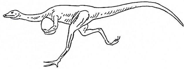
Oviraptor
